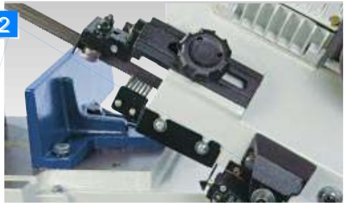
Micro fine taglio, spazzola asportatrucioli - Automatic stop, blade chip brush
